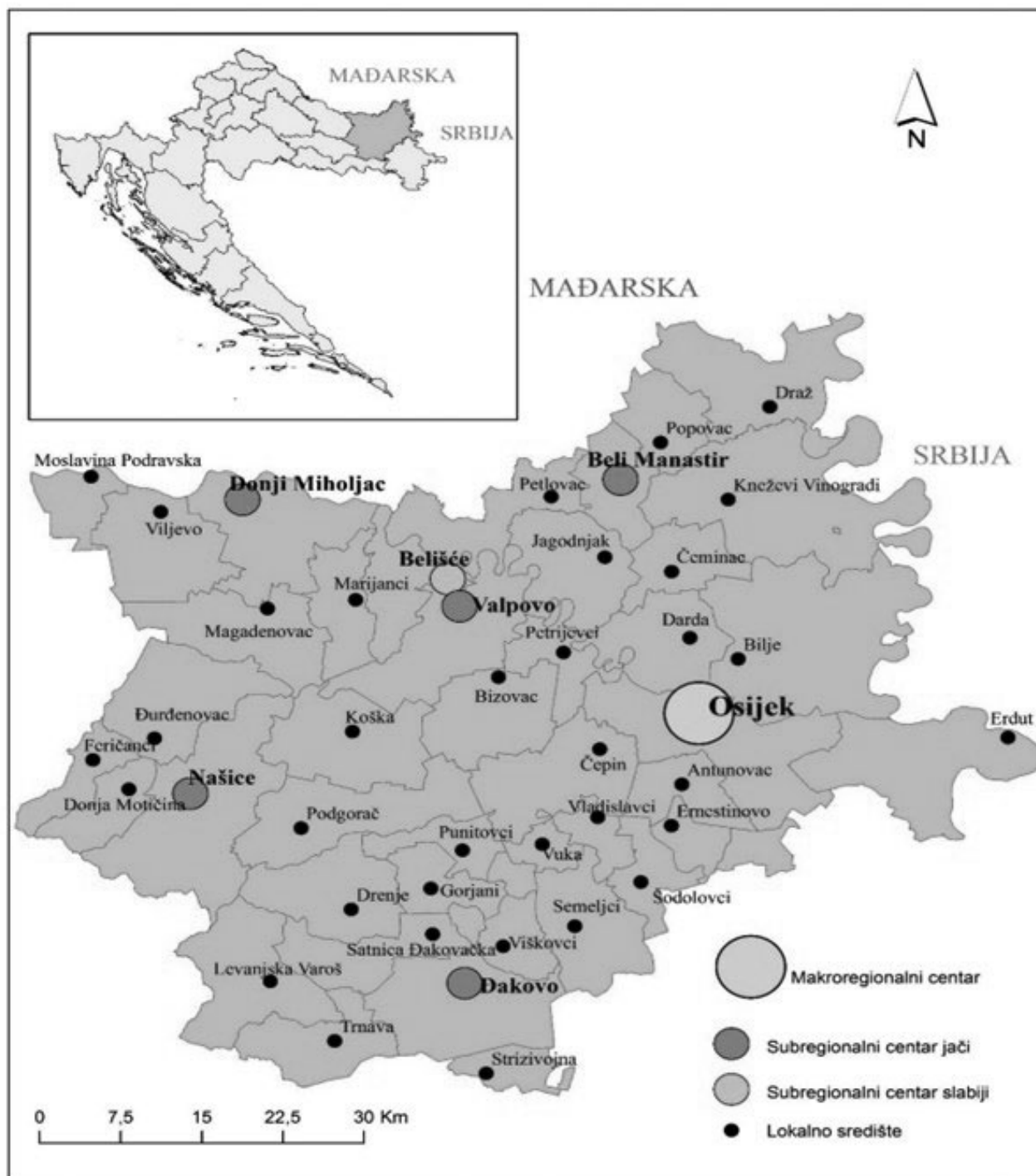
Slika 2.1. Geografski smještaj i upravna organizacija Osječko-baranjske županije
