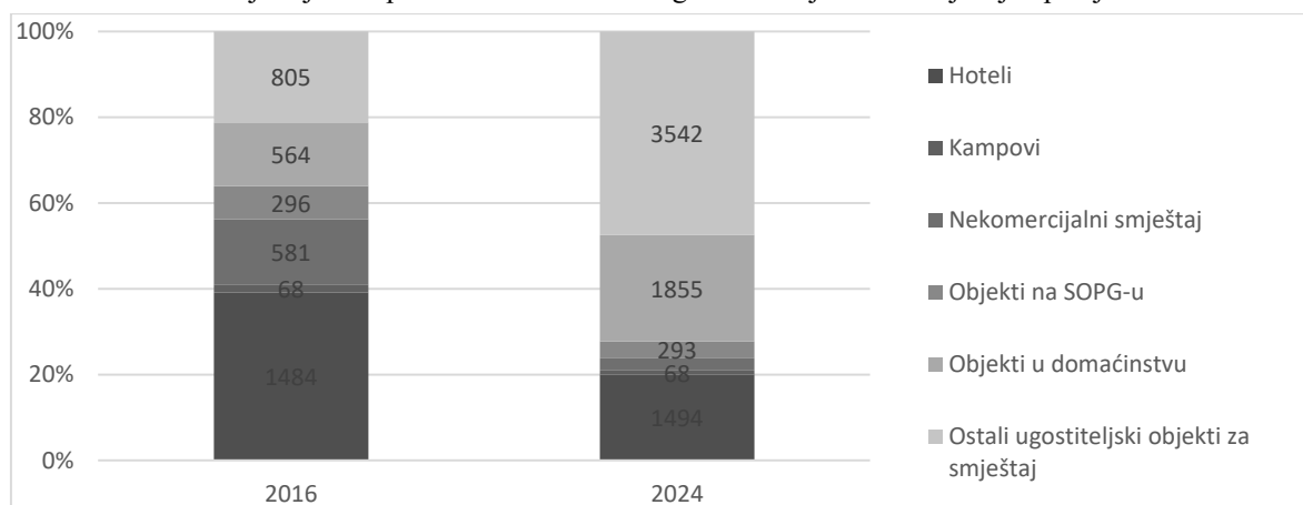
Slika 3.2.2. Udio smještajnih kapaciteta u 2016. i 2024. godini u Osječko-baranjskoj županiji
