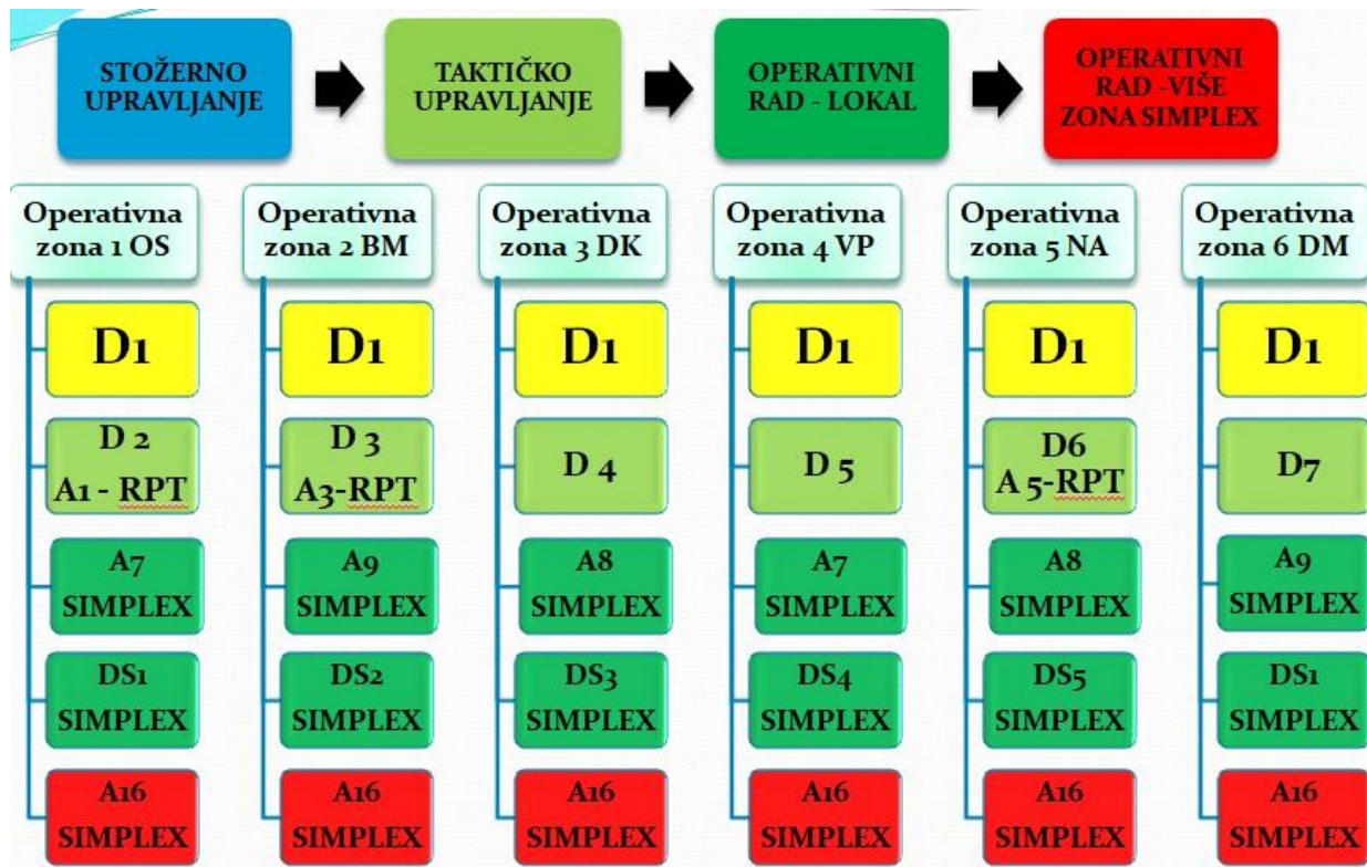
Slika 10.1 – Raspored kanala s uređajima
